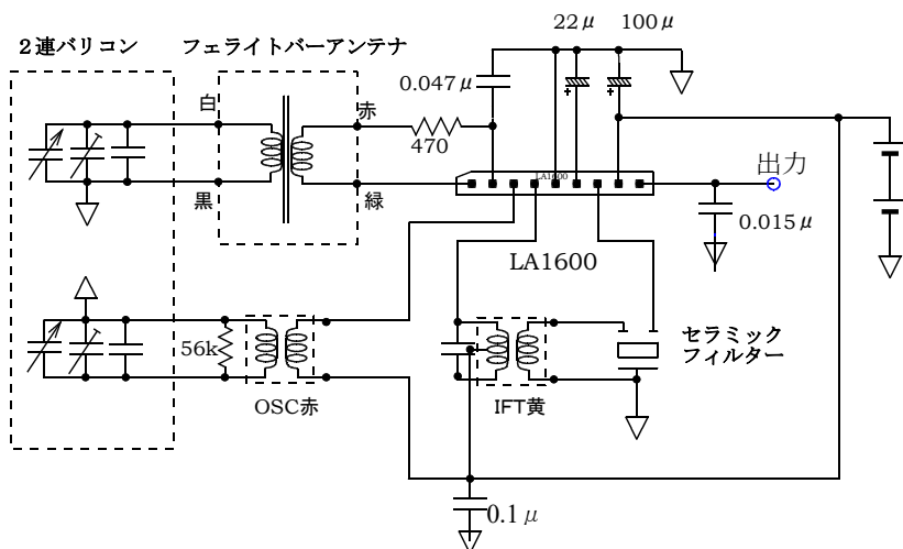
高周波回路
