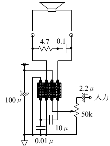
低周波回路
