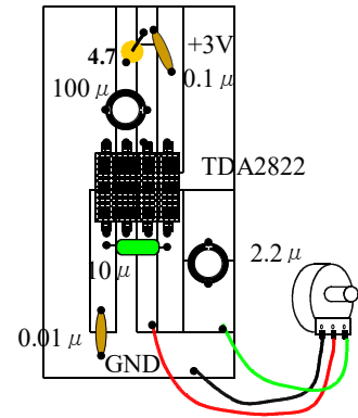
低周波回路 実体配線図
