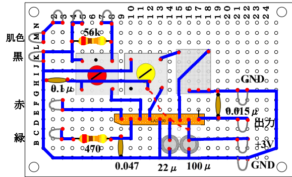
半田面より見た図
